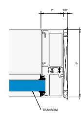
12 Callout - Door - Thermal Transom Jamb B 6" = 1'-0"
