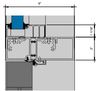
16 Callout - Door - Thermal Transom Head 6" = 1'-0"
