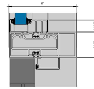
17 Callout - Door - Thermal Transom Head - CoC 6" = 1'-0"
