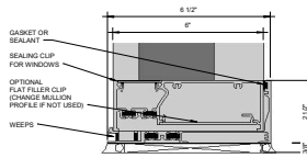
12 Callout - Window Sill 103A - OG 6" = 1'-0"
