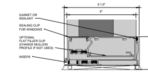
14 Callout - Window Sill 103A - IG 6" = 1'-0"
