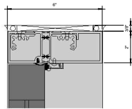
14 Callout - Door - Thermal Head 6" = 1'-0"
