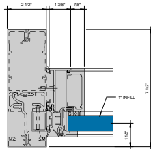
④ LEFT JAMB PO - 1\"/>
