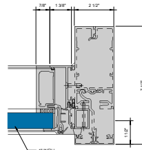
⑤ RIGHT JAMB PO - 1\"/>
