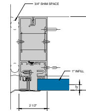
⑦ SSG JAMB - 1" JAMB 6" = 1'-0"
