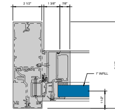
⑥ LEFT JAMB COS - 1\"/>
