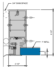
⑤ SGT JAMB - 1" INFILL 6" x 1'-0"
