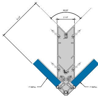
⑤ SGT JAMB - 1" INFILL 6" x 1'-0"
