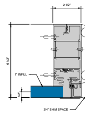
⑦ SGT JAMB - 1" INFILL 6" x 1'-0"
