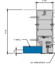
⑦ SGT JAMB - 1" INFILL 6" = 1'-0"
